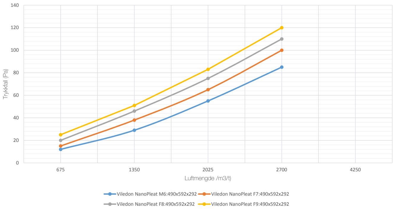
Trykkfall Viledon NanoPleat 490x592x292
